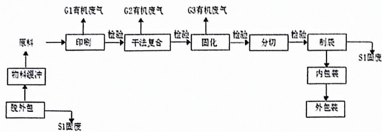
总工艺流程图
