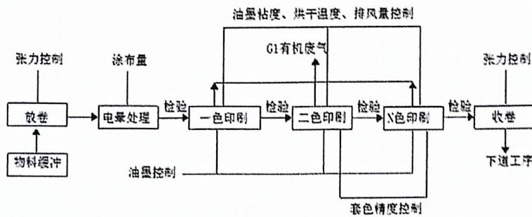
印刷工序工艺流程图
